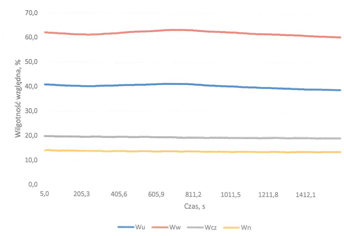
Wyk.2. Przebieg zmian wilgotności powietrza dla serii pomiarowej nr 1.
