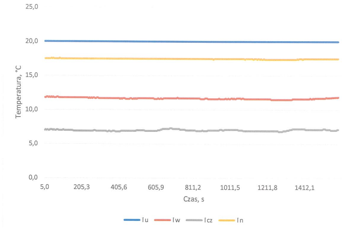
Wyk.1. Przebieg zmian temperatur powietrza dla serii pomiarowej nr 1.
